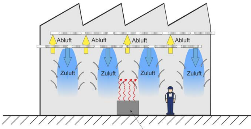
Abb. 6 Prinzip Mischströmung
