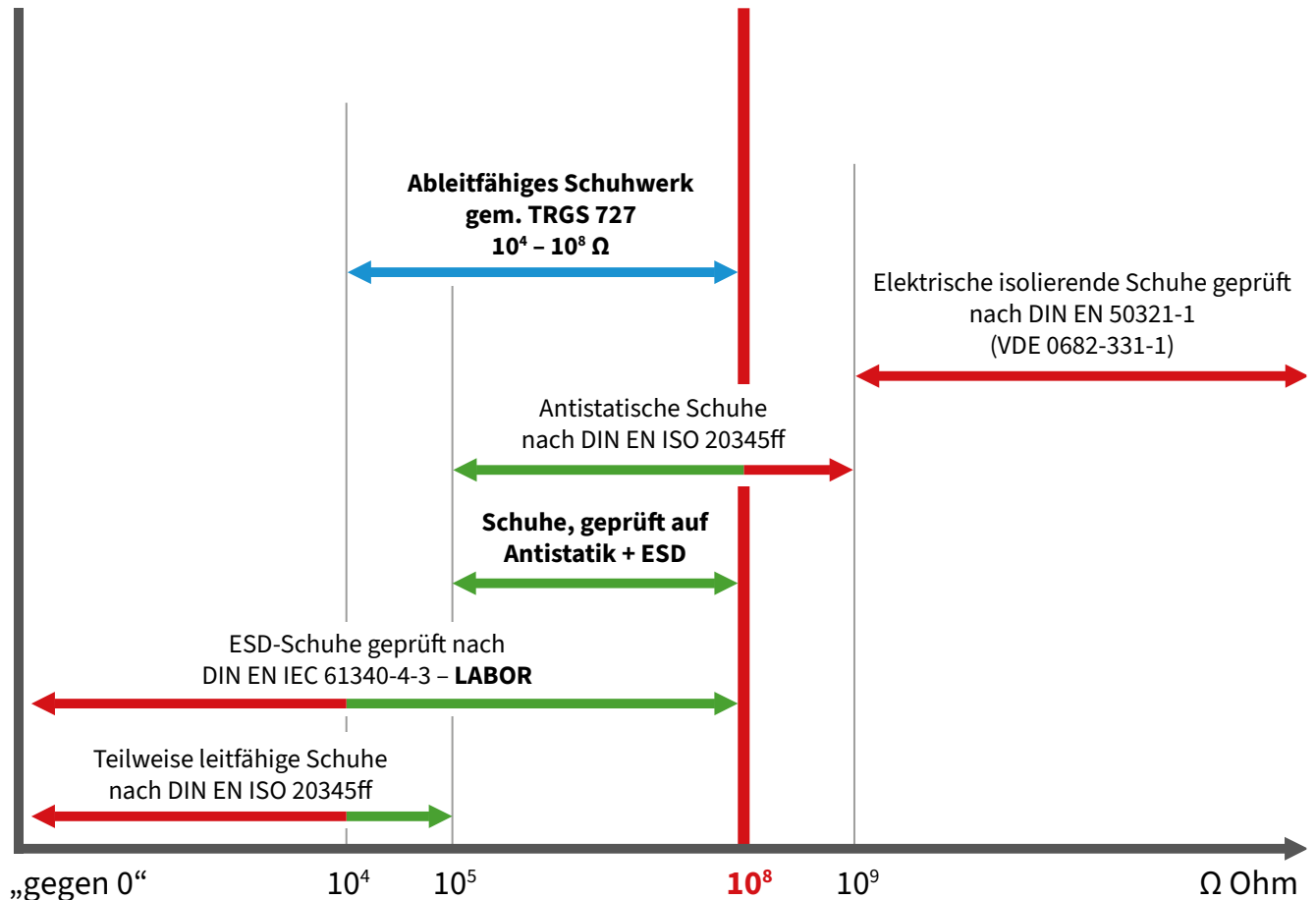
Abb. 29 Schuhtypen und deren elektrische Widerstände
