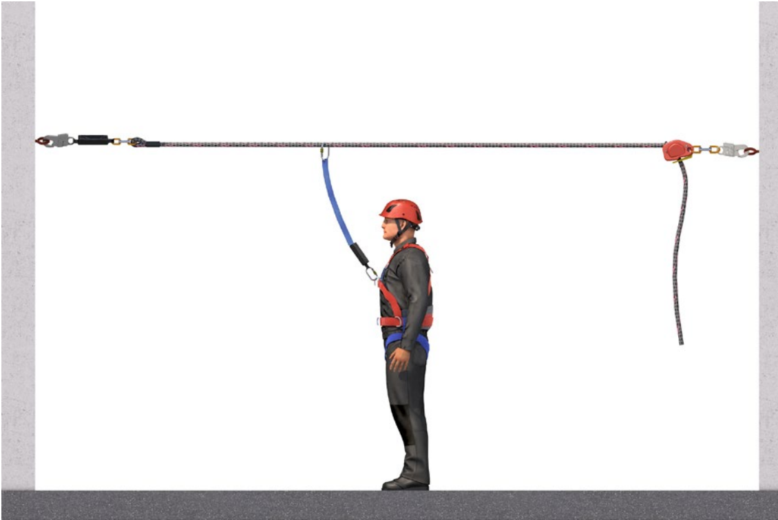
Abb. 66 Skizze einer nicht dauerhaft befestigten Anschlagseinrichtung vom Typ C DIN EN 795 (LifeLine)
