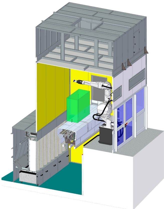
Abb. 36 Spritzlackierautomat
