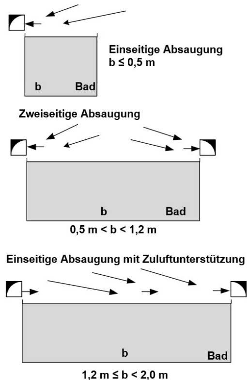
Abb. 43 Absaugeinrichtungen an Taackbehältern
