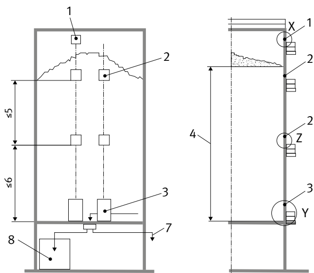
Abb. 8.7 Anordnung von Stocher-Öffnungen über die Silohöhe
