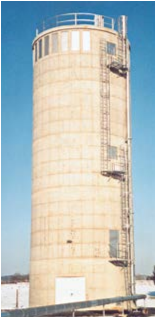
Abb. 5.12 Steigleiteraufstieg mit Wechelpodesten
