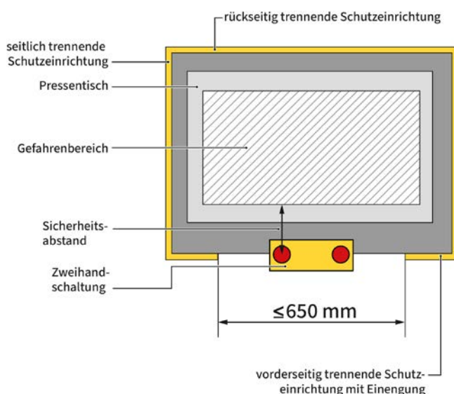
Abb. 28 Werkzeugeinbauraum – Absicherung einer neuen/neueren Metall-Kaltpresse mit ZHS und trennenden Schutzeinrichtungen
