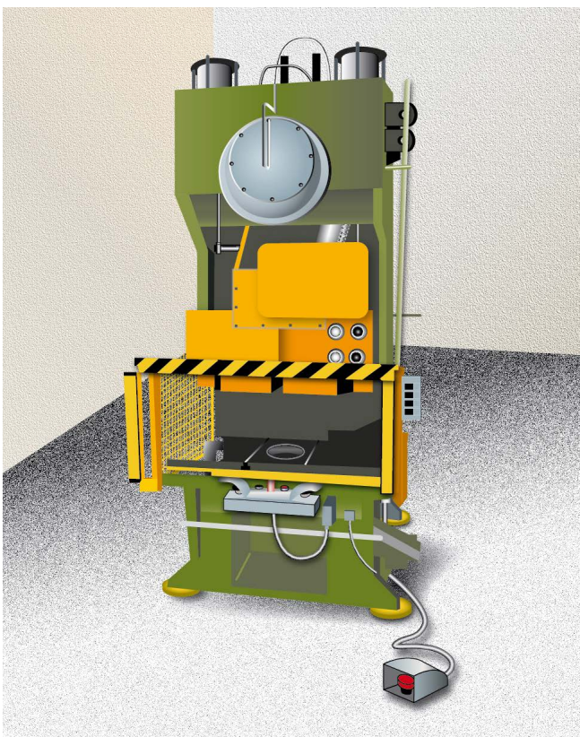
Abb. 3 Exzenterpresse, Antrieb
