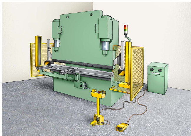
Abb. 6 Hydraulische Gesenkbiegepresse
