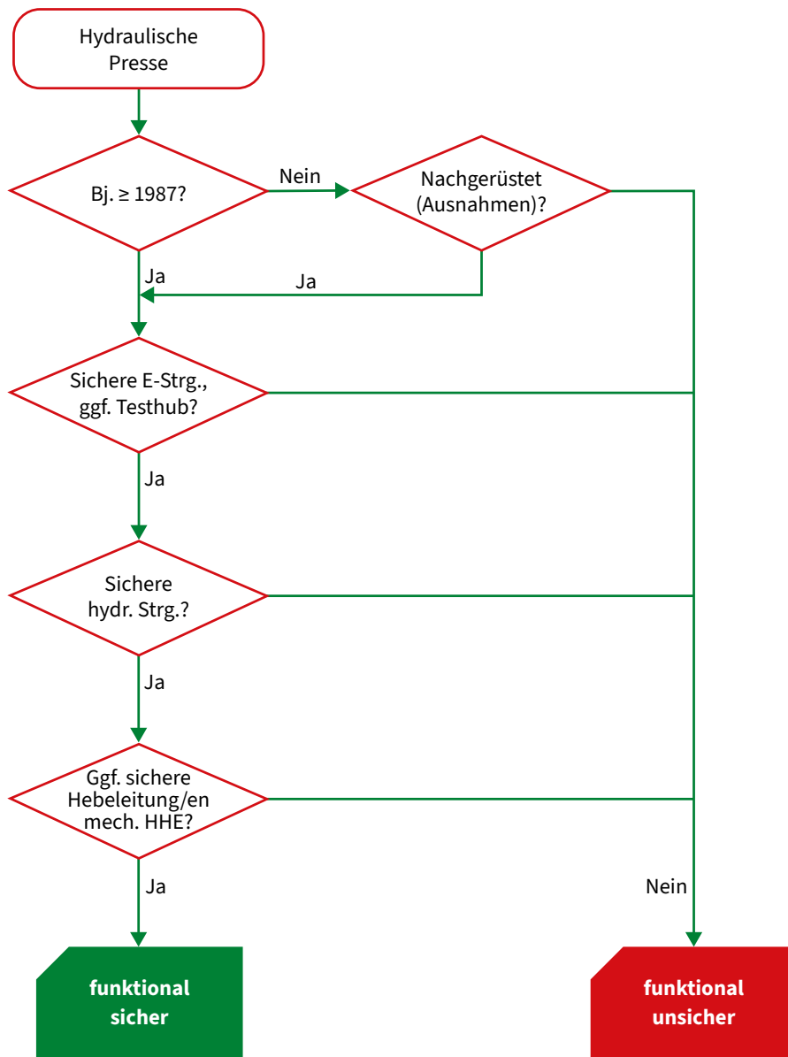
Abb. 17 Entscheidungsschritte – funktional sichere Hydraulikpresse (Mech. HHE: Mechanische Hochhalteeinrichtung)
