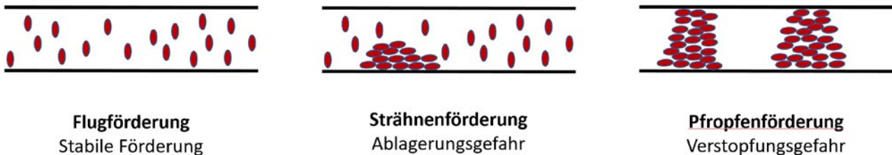
Abb. 3.3.3 Arten der Förderung von Stoffen in Rohrleitungen
