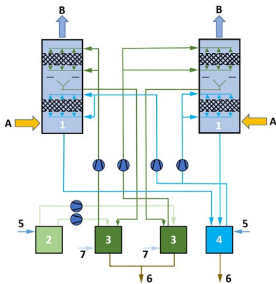
Abb. 3.5.11 Biologische Gaswäsche in einer Metallgießerei als schematische Darstellung
