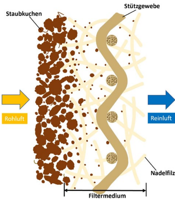
Abb. 3.5.7 Abscheidemechanismen bei Faserschichtfiltern (oben) und Querschnitt eines mit Staub belegten Filtermediums (unten), Prinzipskizzen [30]
