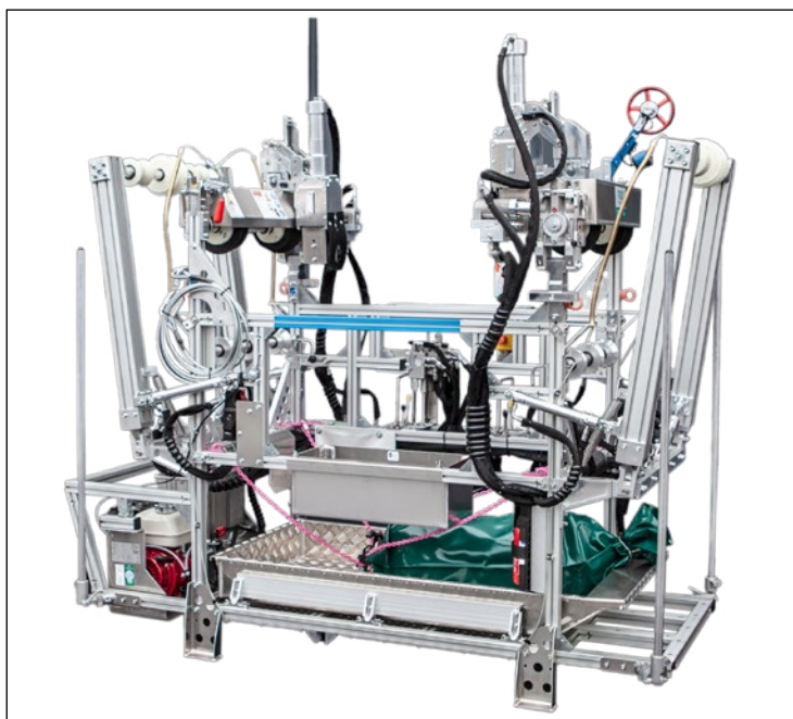
Abb. 120 Beispiel für ein Leitungsfahrzeug mit Kraftantrieb.
