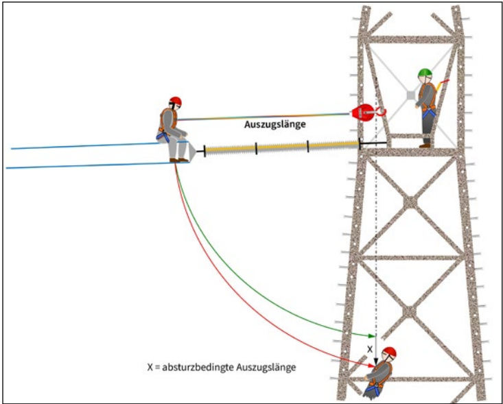
Abb. 54 Schematische Darstellung der Gefährdungen durch einen Pendelsturz beim Übersteigen von Abspannketten.
