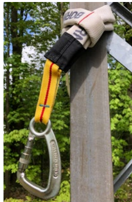
Abb. 58 Beispiel einer speziellen Bandschleife für erhöhte Belastungen. Im Belastungsfall können Bandschlingen durch Scherkräfte in Konstruktionsteilen übermäßig belastet werden. Es empfiehlt sich daher ein Einsatz speziell für diese Benutzung ausgewiesener Schlaufen.
