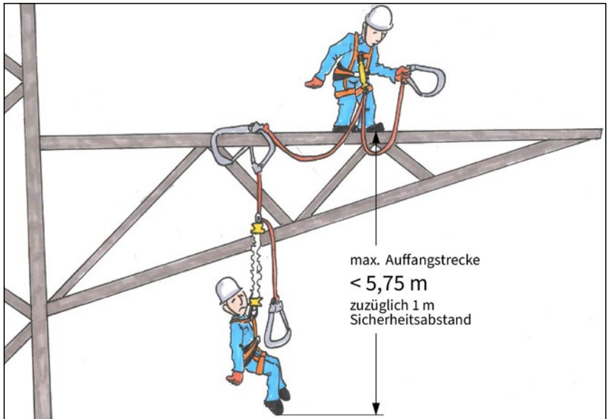
Abb. 28 Absturz von einer Harfentraverse mit einem Anschlagpunkt auf Fußniveau. Die normativ maximale Auffangstrecke beträgt < 5,75 m.
