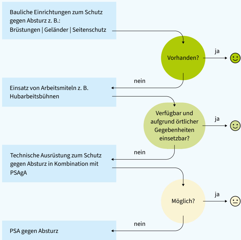
Abb. 1 Systematik der Schutzmaßnahmen gegen Absturz.
