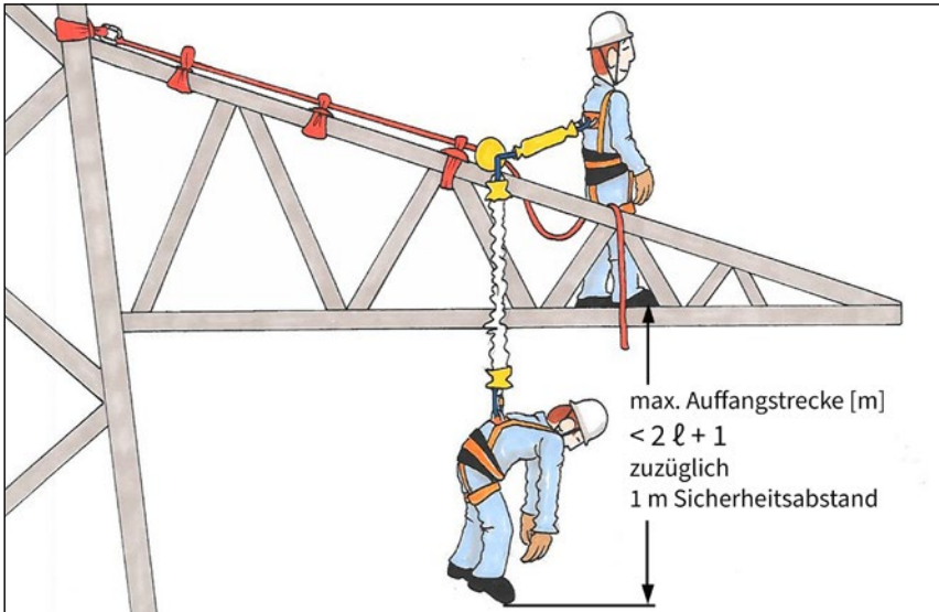
Abb. 25 normativ maximale Auffangstrecke bei einem Absturz von einer Traverse in ein mitlaufendes Auffanggerät einschließlich beweglicher Führung. Gemäß EN 353-2 beträgt „l“ max. 1 m. Der Abstand der Zwischensicherungen sollte 2 m nicht überschreiten, um Pendelsturz und Auffangstrecke zu minimieren.
