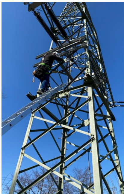
Abb. 82 Die Verwendung der üblichen Masthängeleitern als Zugangsweg zum Eckstiel bietet hier ein hohes Maß an Sicherheit, da durch die Einhängebügel weder ein seitliches Verrutschen noch ein „Absacken“ aufgrund der Bodenbeschaffenheit möglich ist.
