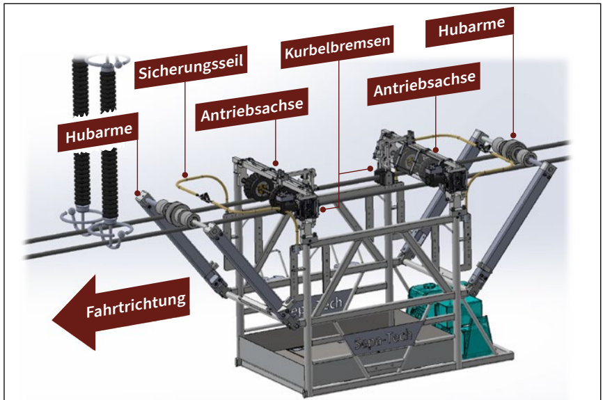
Abb. 131 Leitungsfahrzeug (LTF) vor dem Überfahren von Tragketten-Hubarme, Sicherungsseile und Antriebsachsen sind geschlossen.
