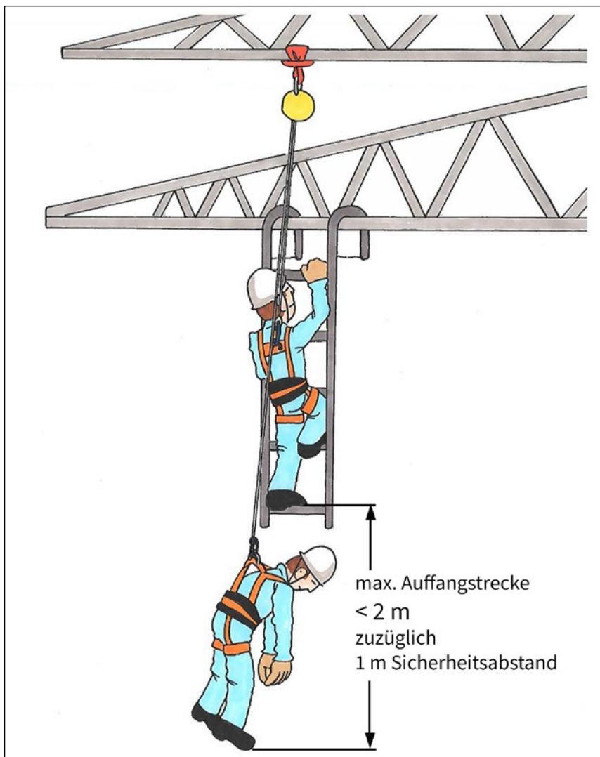
Abb. 30 Beispiel für den Einsatz eines Höhensicherungsgeräts beim Besteigen einer Hängeleiter mit Angabe der normativ zulässigen Auffangstrecke.
