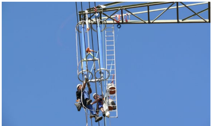
Abb. 48 Beispiel für ein HSG mit einem Drahtseil-Verbindungsmittel.
