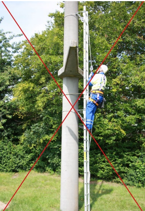
Abb. 88 Beispiel für eine Maststeigleiter ohne feste Führung.
