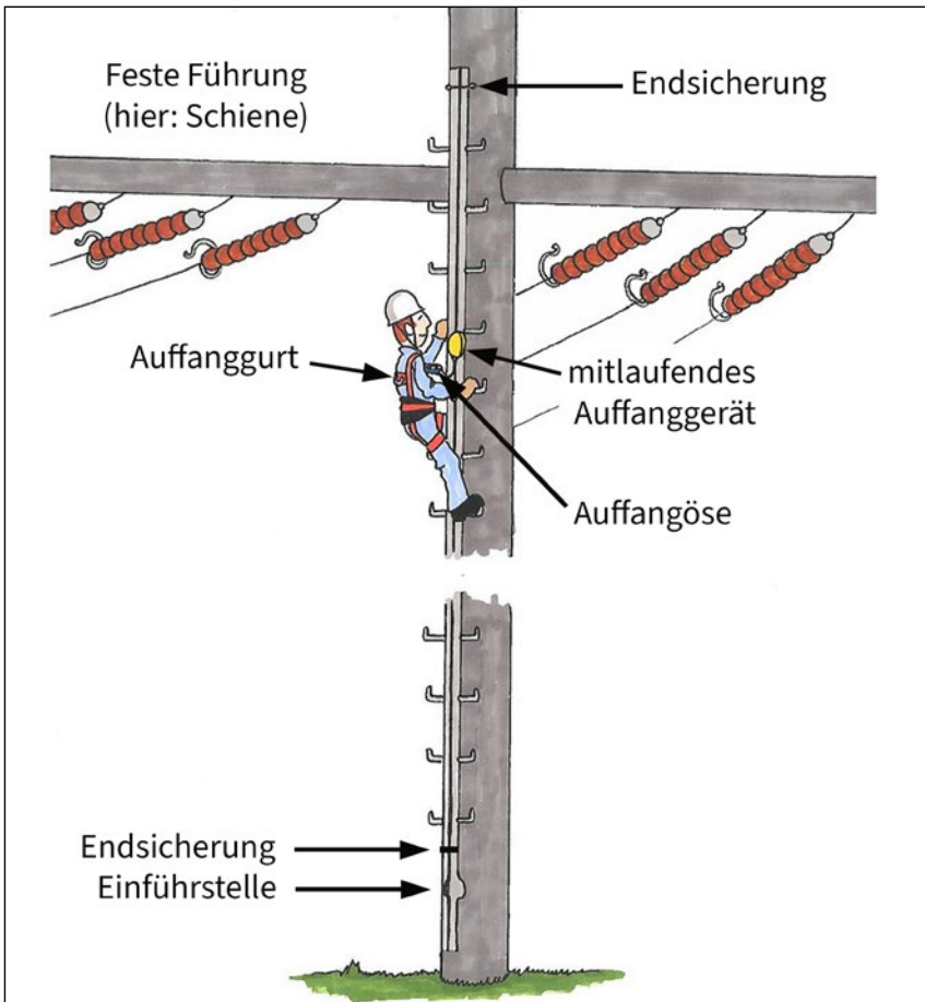
Abb. 21 Auffangsystem mit einem mitlaufenden Auffanggerät einschließlich fester Führung. Feste Führungen können als Schienensysteme oder als gespannte Stahlseile ausgeführt sein. Die Sicherung erfolgt über ein mitlaufendes Auffanggerät, das mit der zugehörigen Auffangöse des Auffanggurtes verbunden ist.
