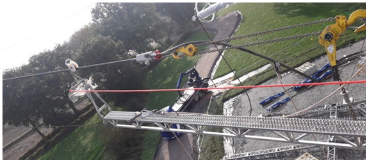
Abb. 110 Die mit der Traverse verbundene Bühne wird in die Arbeitsposition gezogen und am Leiterseil eingehängt.
