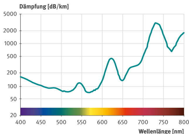
Abb. A3.8 Dämpfungsverlauf der Polymer-Optischen-Faser (Quelle: POF-AC)
