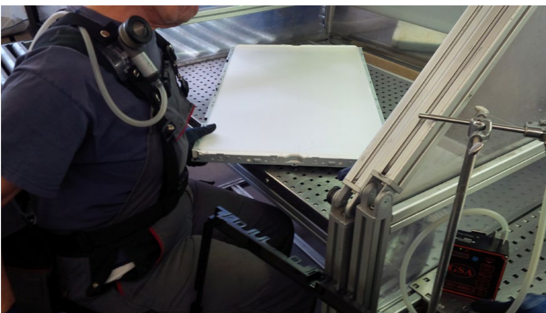
Abb. 2 Demontagearbeitsplatz (abgesaugt), Quecksilbermessung an der Person
