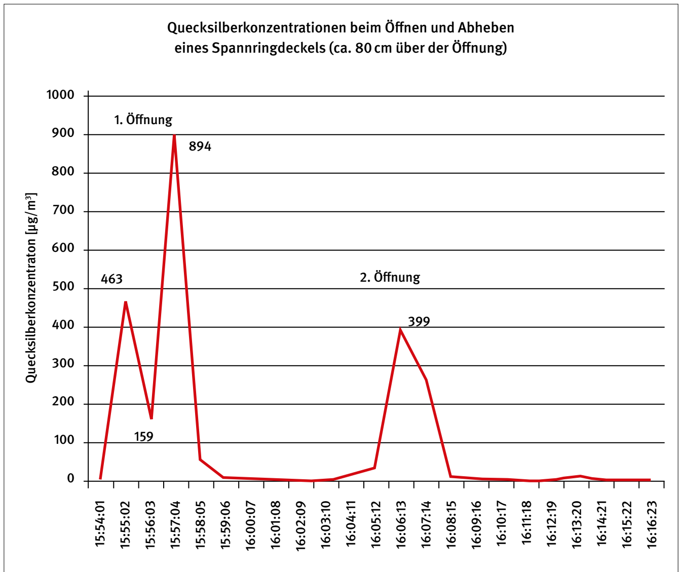
Abb. 6 Quecksilberkonzentration beim Öffnen eines Bruchbehälters mit Glasbruch – vertikal Abheben des Spannringdeckels nach oben zum Einfüllen von Glasbruch
