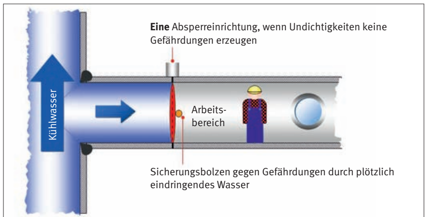
Abb. 8.2.1 Als wirksame Absperrmaßnahme genügt eine Absperrvorrichtung, wenn Versicherte bei Undichtigkeiten nicht gefährdet werden können. Absperrvorrichtungen sind mit Sicherungsbolzen auszuführen, wenn Gefährdungen durch plötzlich eindringendes Wasser gegeben sind.
