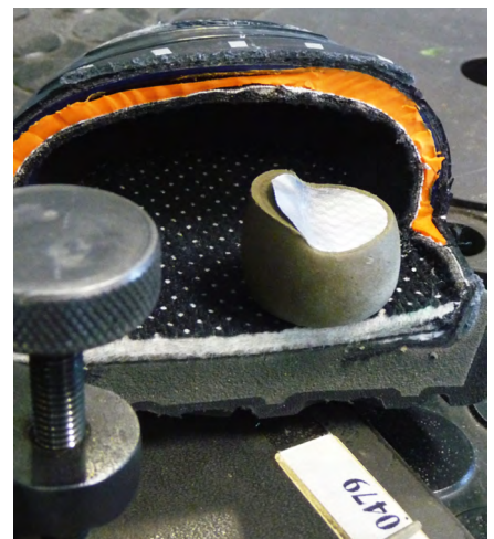
Zehenschutzkappen und Prüfkörper nach der Druckprüfung
