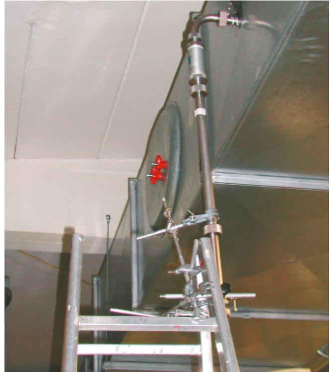
Abb. 8: IPS in der Abluft einer RLT-Anlage
