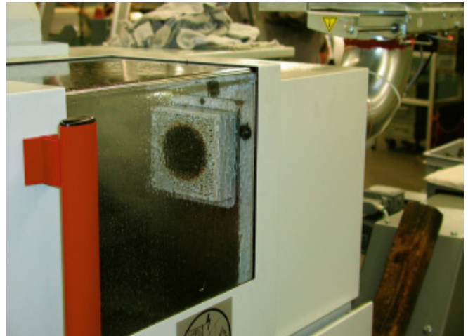
Abb. 23: Tropfenabscheider vor der Ansaugöffnung zur Minimierung des KSS-Verlustes aus der Maschine
