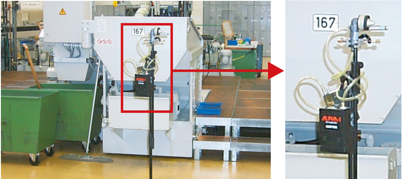
Abb. 1 und 2: Stationäre Probenahme mit PAS-Pumpe, Aktivkohleröhrchen und Gesamtstaub-Gas-Probenahmesystem (GGP), Mess- und Analyseverfahren sind detailliert in der BGIA-Arbeitsmappe „Messung von Gefahrstoffen“ unter der Kennzahl 7750 veröffentlicht.
