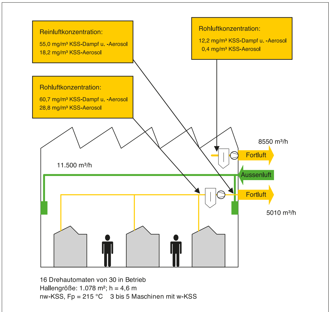
Abb. 15: Skizze zum Hallenlüftungskonzept 3, Betrieb C
