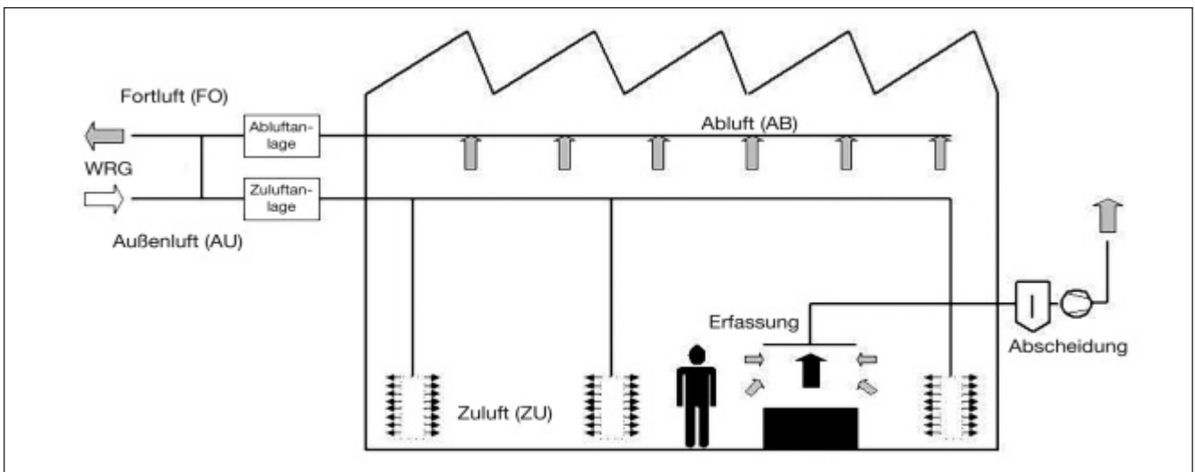
Abb. 24: Empfohlenes Lüftungskonzept mit Schichtlüftung und Fortluft
