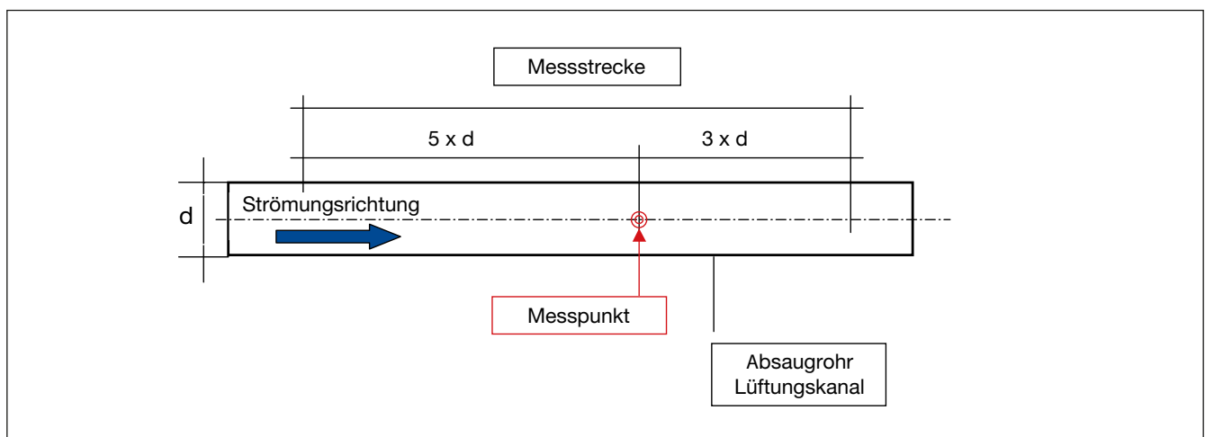
Abb. 5: Messstrecke in Rohrleitungen und Lüftungskanälen
