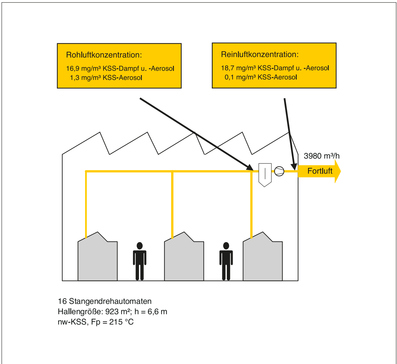
Abb. 9: Skizze zum Hallenlüftungskonzept 1, Betrieb A
