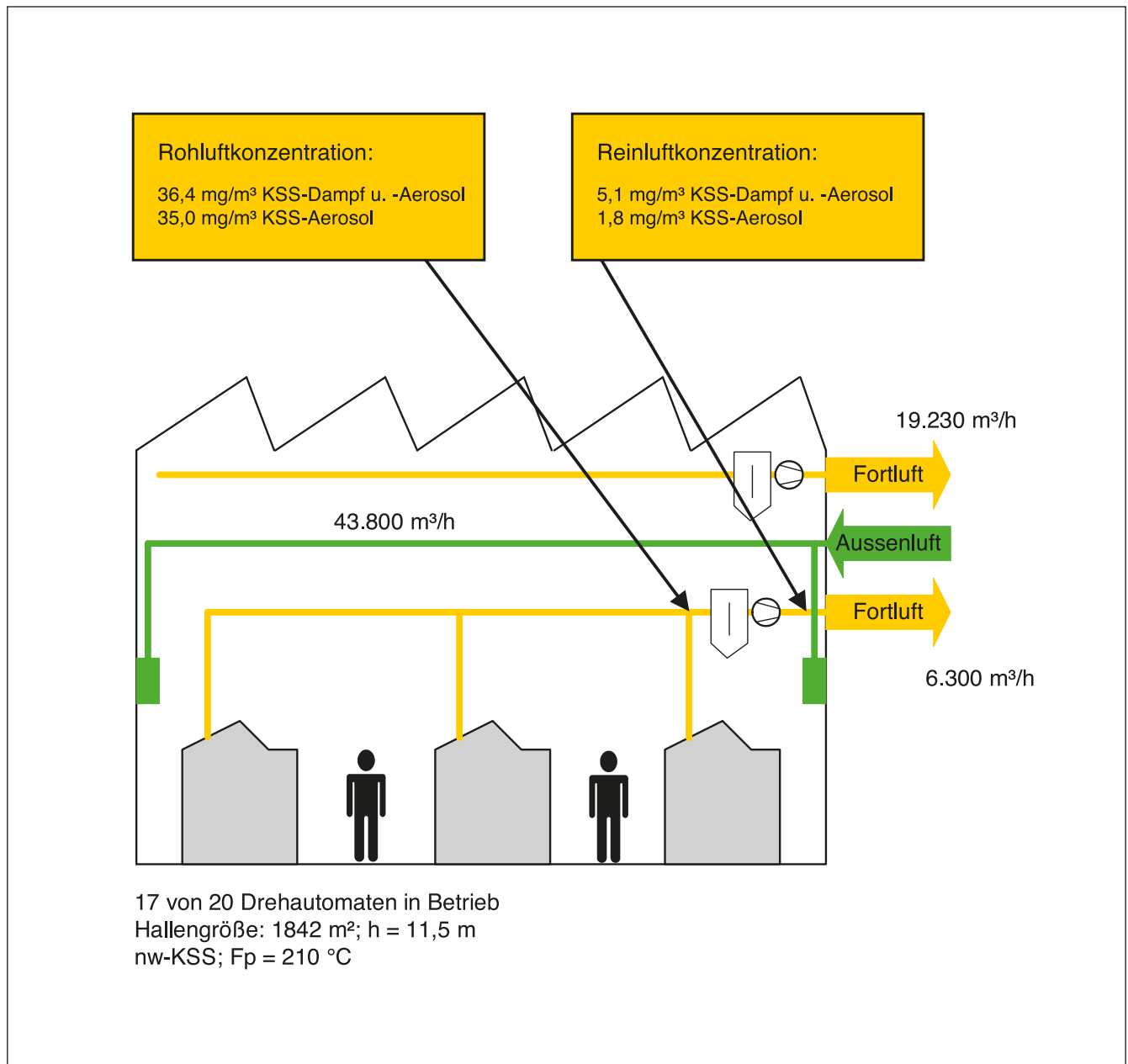
Abb. 18: Skizze zum Hallenlüftungskonzept 3, Betrieb D
