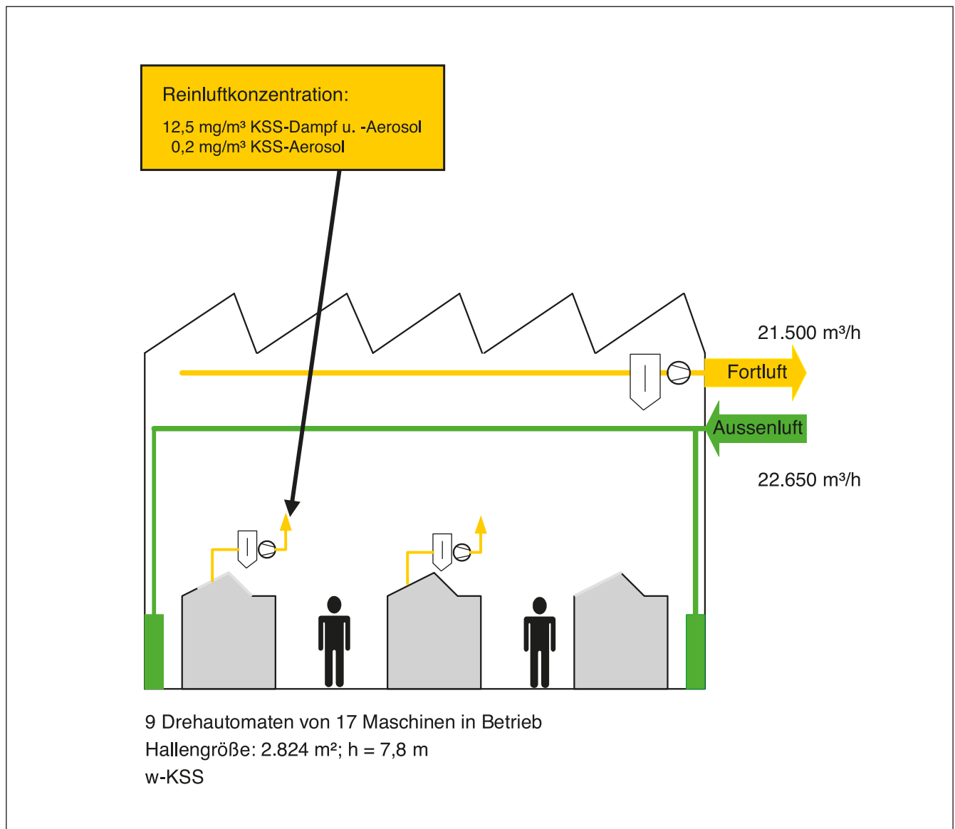
Abb. 12: Skizze zum Hallenlüftungskonzept 2, Betrieb B
